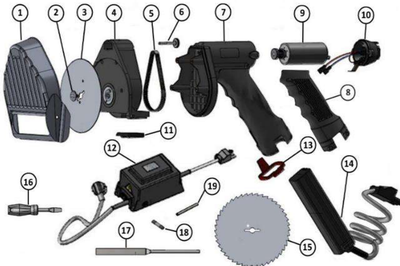
Explosionszeichnung- JET 120 Delux 70 Watt
